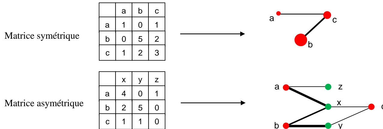
Figure 1 : Représentations graphiques d'une matrice symétrique et d'une matrice asymétrique
